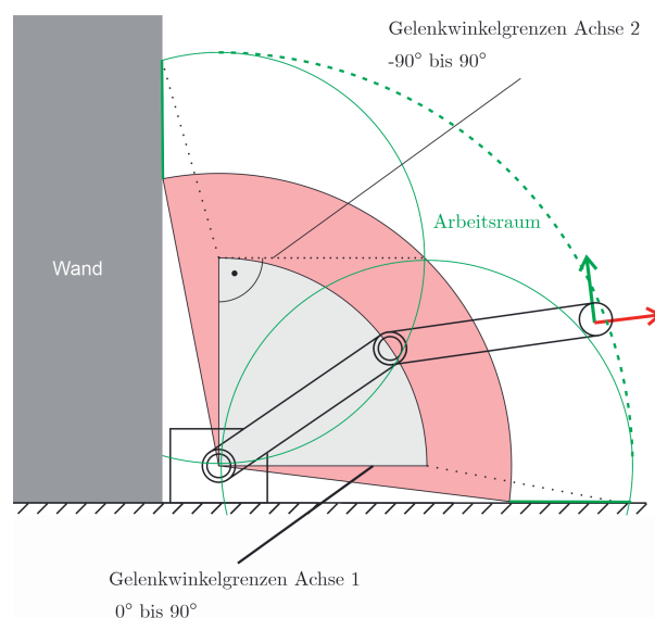
Abbildung 11: Arbeitsraum eines Roboters
