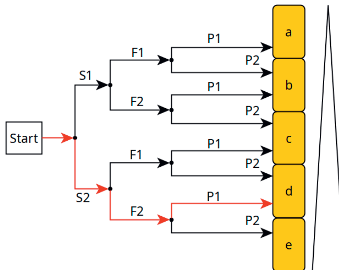
Abbildung 3: Risikograph nach DIN13849-1 zur Ermittlung des PL_r . Der Pfeil rechts gibt eine abnehmende Schwere des Risikos von unten nach oben an.
