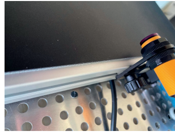
Abbildung 39: Befestigung der Lichtschanke an der Gewindeplatte des Förderbandes
